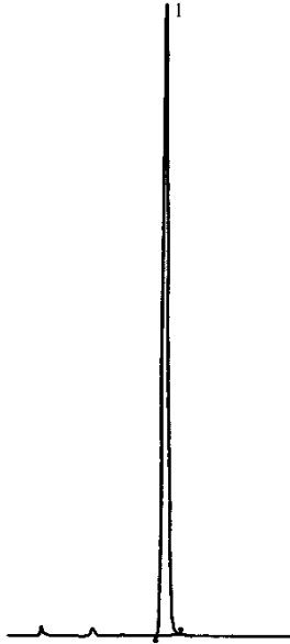
图 2 福美双原药的高效液相色谱图
