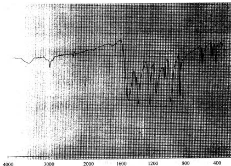
图 1 福美双标样的红外光谱图
